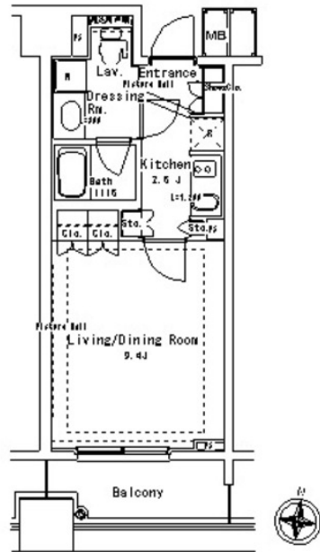
間取り図
